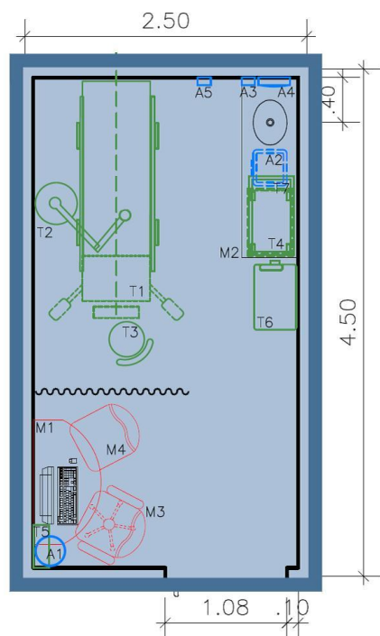
PLANTA BAIXA
