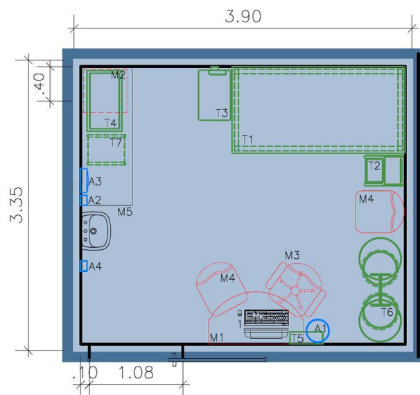
PLANTA BAIXA
