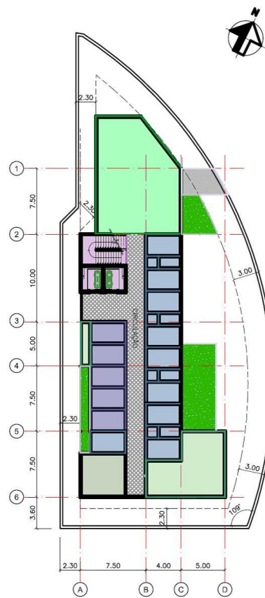
PLANTA PAV. SUPERIOR CENTRO DE SAÚDE SANTA MÔNICA
