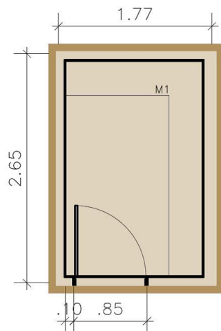
PLANTA BAIXA
