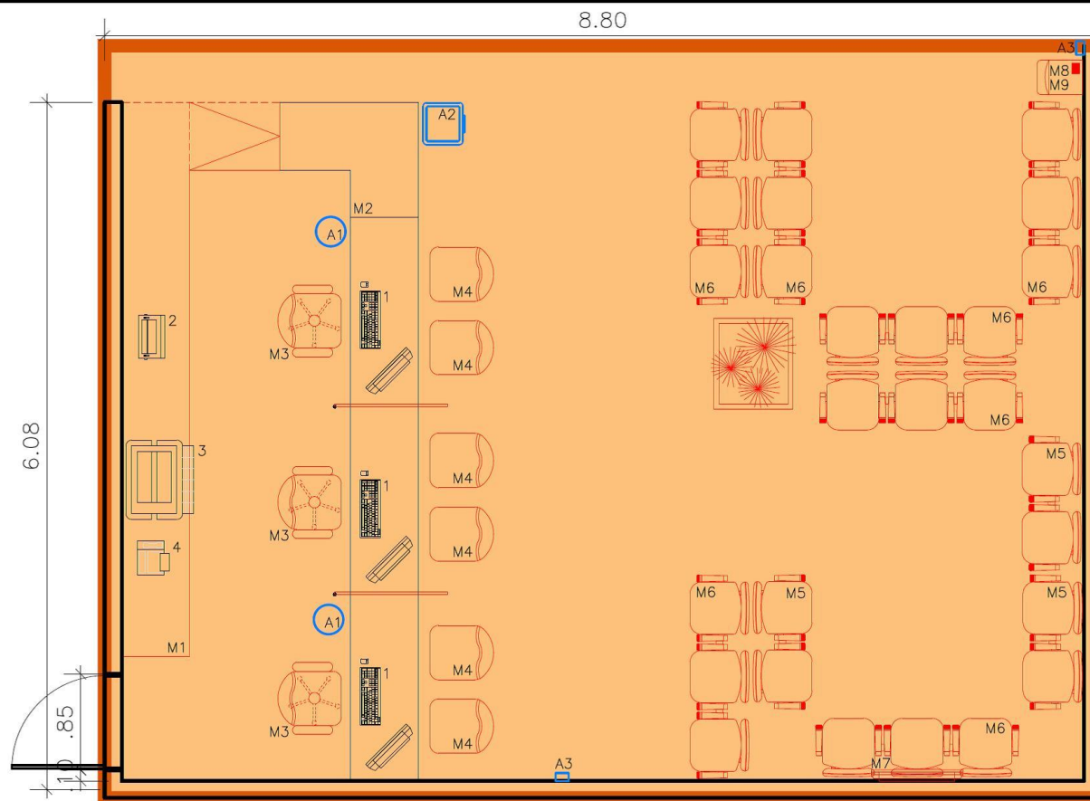
PLANTA BAIXA RECEPÇÃO E ESPERA
