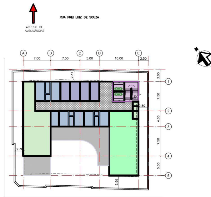
PLANTA PAV. TERREO CENTRO DE SAÚDE JOÃO PINHEIRO
