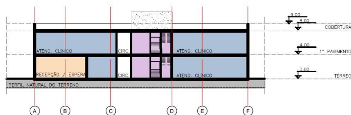
CORTE ESQUEMÁTICO
