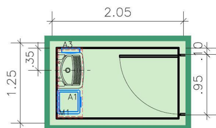
PLANTA BAIXA
