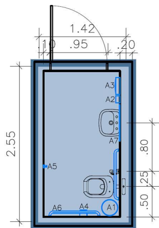
PLANTA BAIXA
