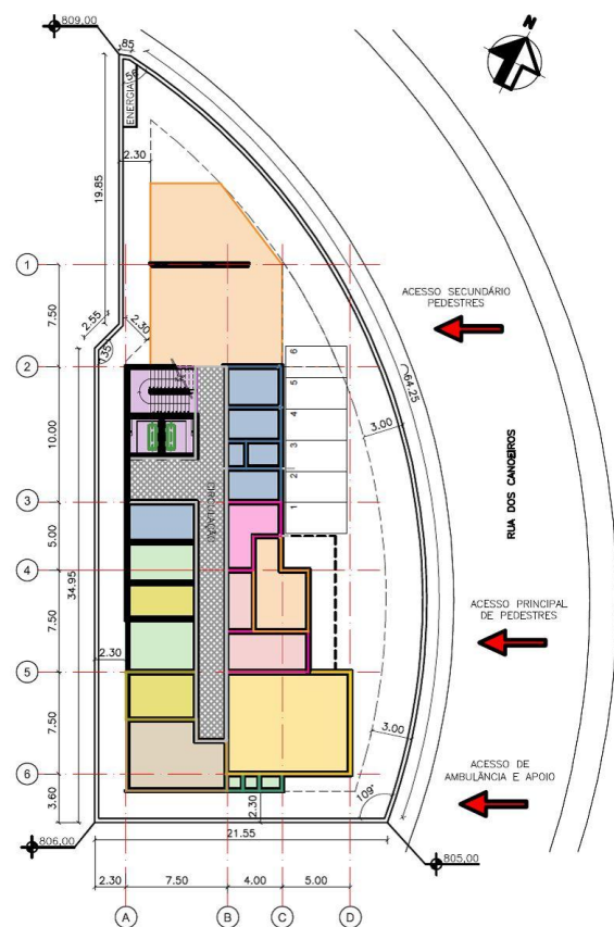
PLANTA PAV. TÉRREO CENTRO DE SAÚDE SANTA MÔNICA
