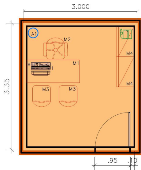
PLANTA BAIXA
