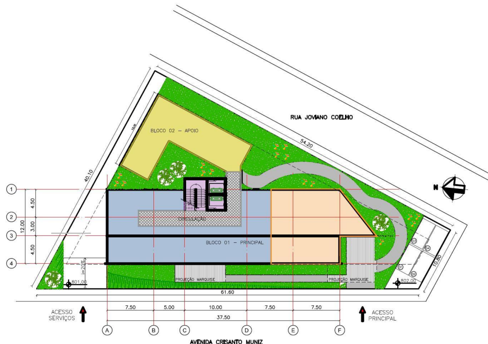
IMPLANTAÇÃO CENTRO DE SAÚDE VISCONDE DO RIO BRANCO
