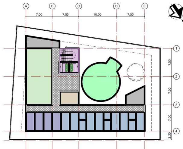
PLANTA PAV. SUPERIOR CENTRO DE SAÚDE SÃO BERNARDO
