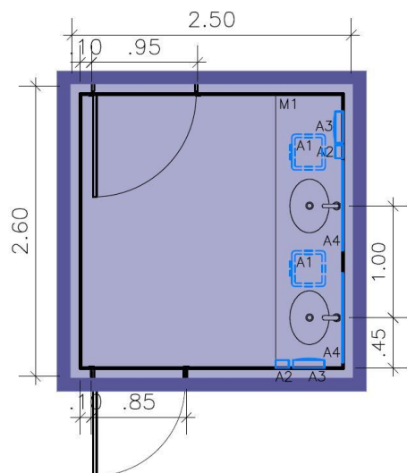
PLANTA BAIXA
