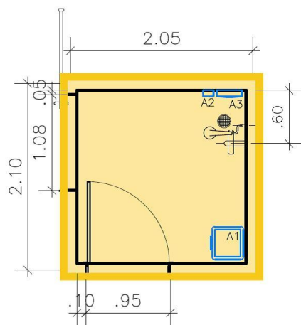
PLANTA BAIXA
