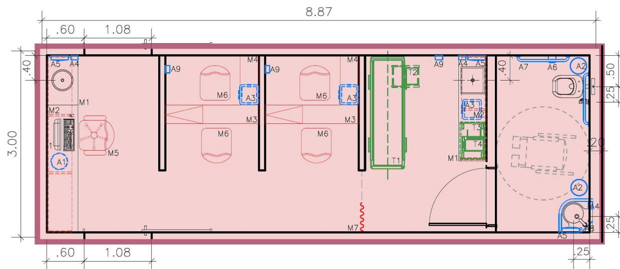
PLANTA BAIXA SALA DE COLETA
