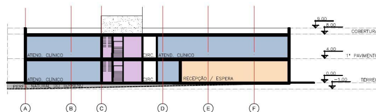
CORTE ESQUEMÁTICO
