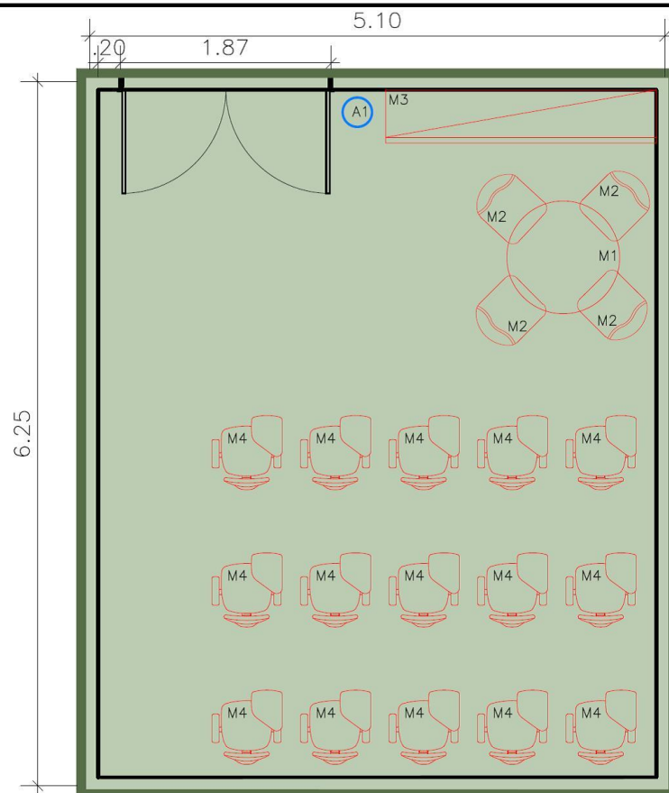
PLANTA BAIXA
