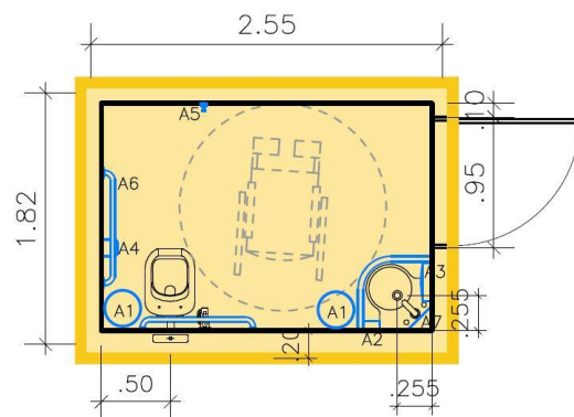
PLANTA BAIXA
