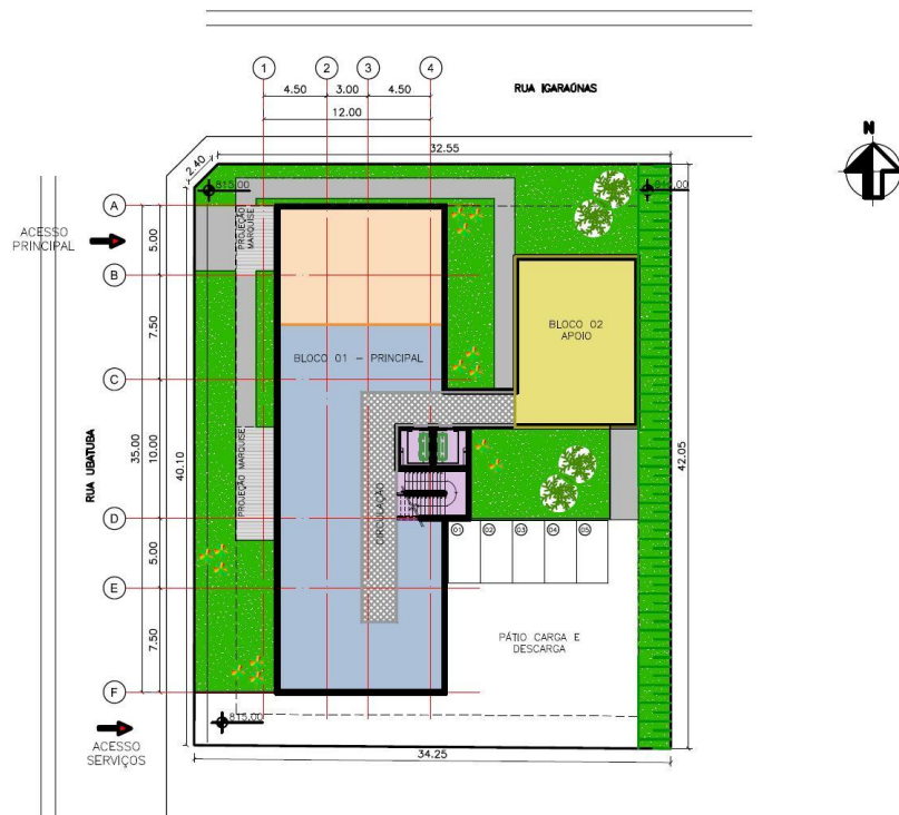
IMPLANTAÇÃO CENTRO DE SAÚDE FLORAMAR 1
