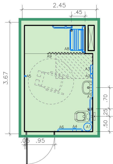
PLANTA BAIXA
