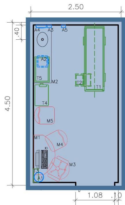
PLANTA BAIXA
