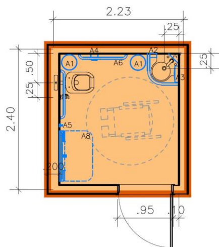
PLANTA BAIXA
