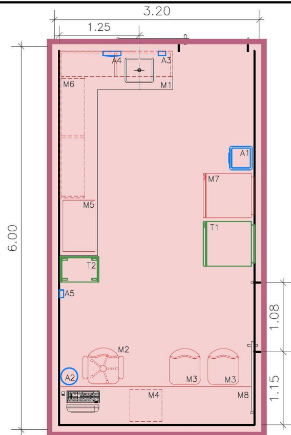
PLANTA BAIXA
