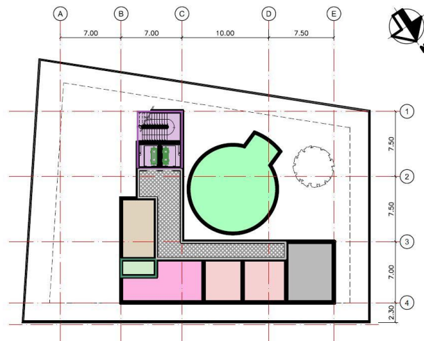
PLANTA PAV. INFERIOR CENTRO DE SAÚDE SÃO BERNARDO
