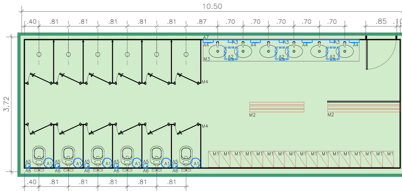
PLANTA BAIXA VESTIÁRIO DE FUNCIONÁRIOS FEMININO
