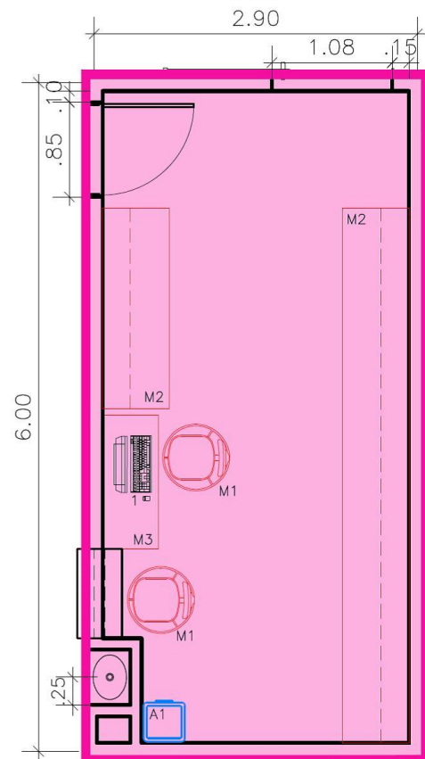
PLANTA BAIXA
