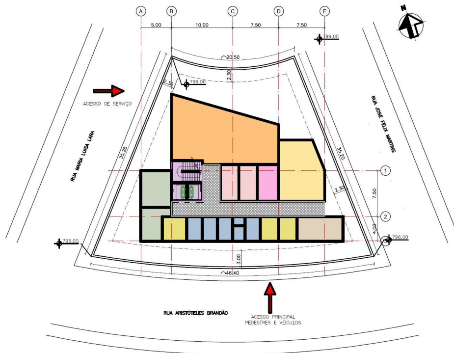
PLANTA PAV. TÉRREO CENTRO DE SAÚDE MANTIQUEIRA
