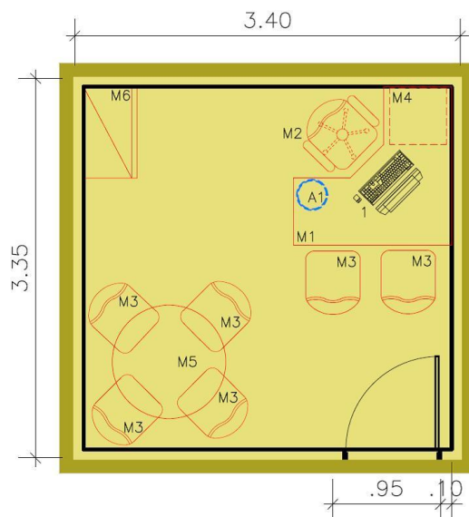
PLANTA BAIXA
