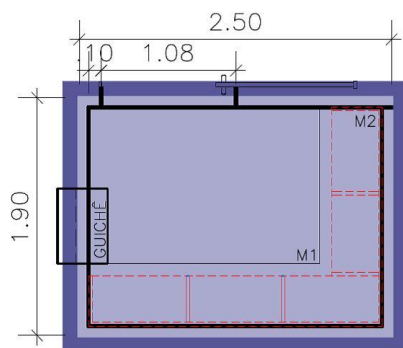
PLANTA BAIXA
