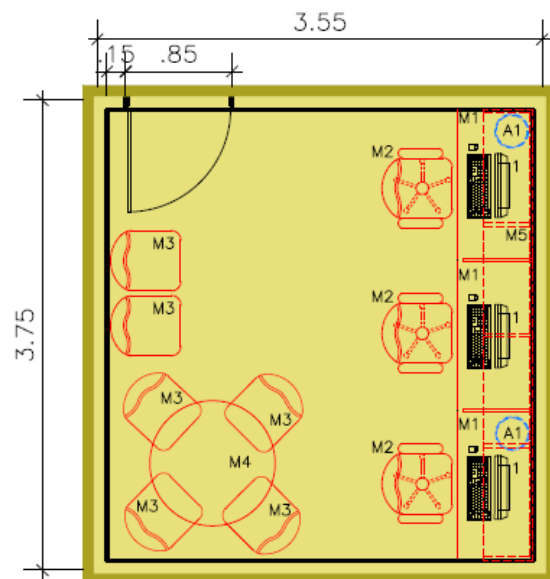
PLANTA BAIXA
